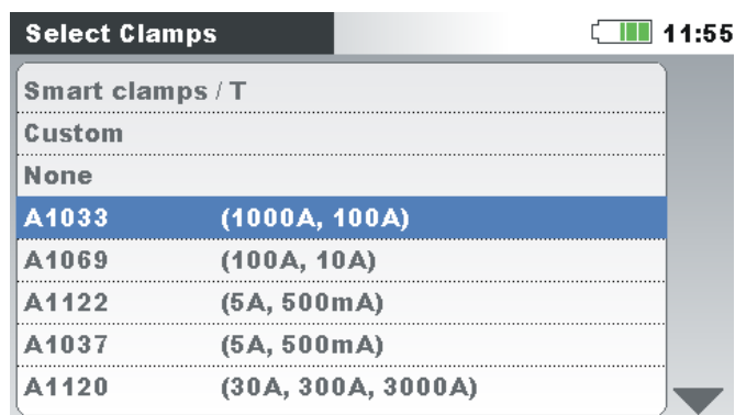
Abbildung 3-5: Stromzangen Auswahl
