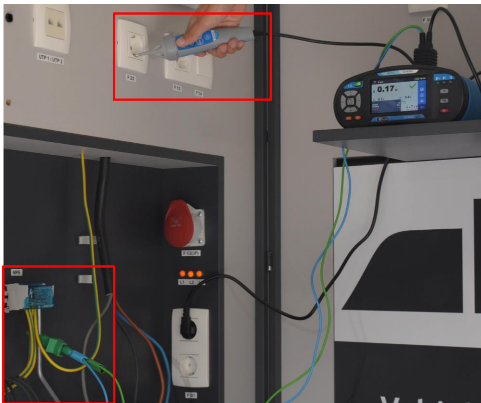
Abbildung 2-42: Durchgangsprüfung zwischen MPE (Hauptpotentialausgleich) und Steckdose
