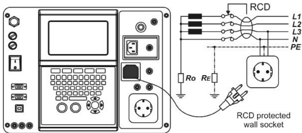
Abbildung 4-36: Prüfung eines RCD in der Elektroinstallation
