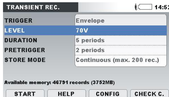
Abbildung 4-85: Einstellungen Transienten-Rekorder
