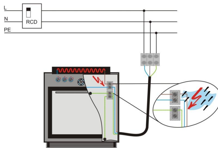
Abbildung 4-26: Funktions- und Ableitstromprobleme
