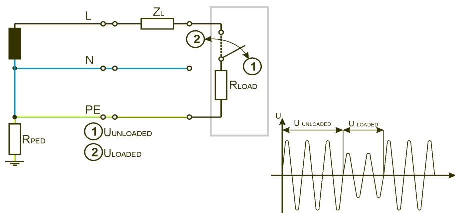
Abbildung 1-7: Schleifenimpedanzmessung - Standardmethode
