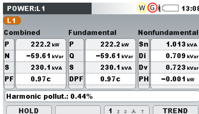
Abbildung 4-54: Kapazitive Last auf Phase L1
