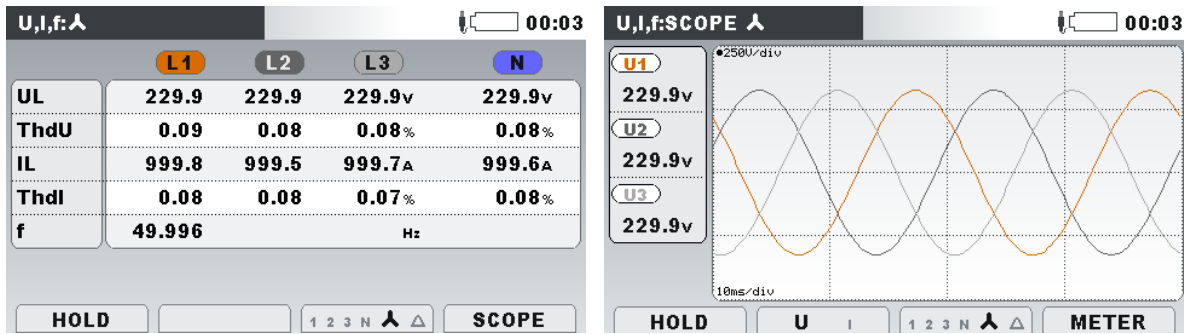
Abbildung 4-91: Echtzeitmessungen von Spannung und Strom
