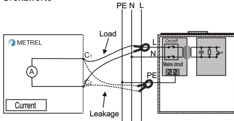
Abbildung 4-27: Beispiele für Prüfungen mit Stromzangen
