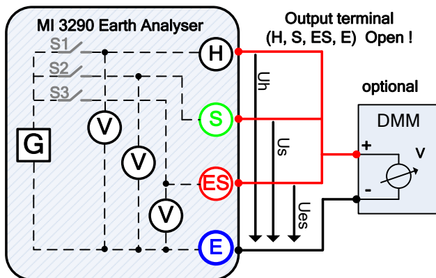
Abbildung 11.98: Beispiel Checkbox (Kontrollkasten) Messungen Volt-Meter
