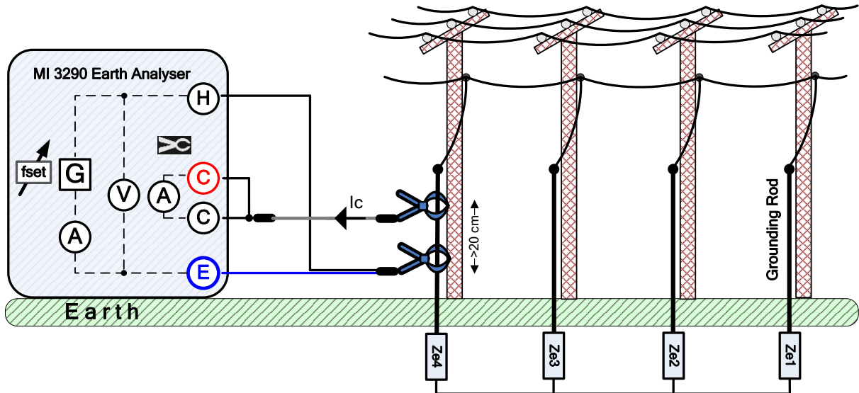
Abbildung 11.24: 2 Stromzangen Messung
