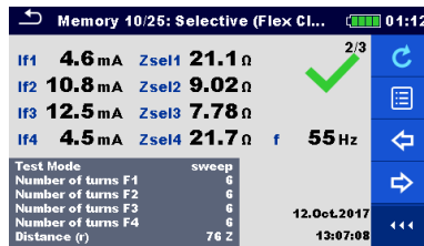
Abbildung 11.34: Beispiel selektive (flexible Stromzangen 1 - 4) Messergebnisse - Z_{sel1-4}
