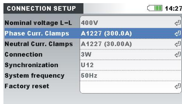
Abbildung 122: Automatisch erkannte Einstellungen für die Stromzangen
