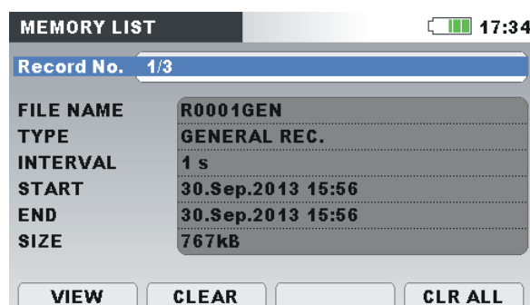
Abbildung 73: Erste Seite der Allgemeinen Aufzeichnung im Menü SPEICHERLISTE
