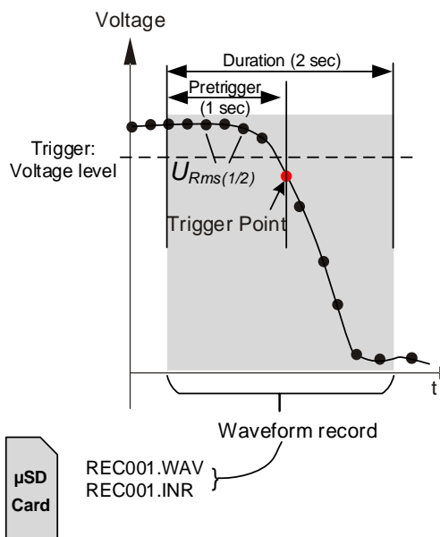
Abbildung 163: Spannungs-Niveau-Auslösung
