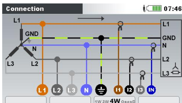
Abbildung 98: Auswählen des 3-Phasen 4-Leitersystems auf dem Gerät
