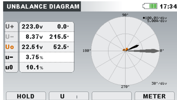
Abbildung 45: Bildschirm mit dem Unsymmetriediagramm
