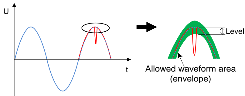
Abbildung 168: Feststellung des Transienten-Auslösers (Hüllkurve)
