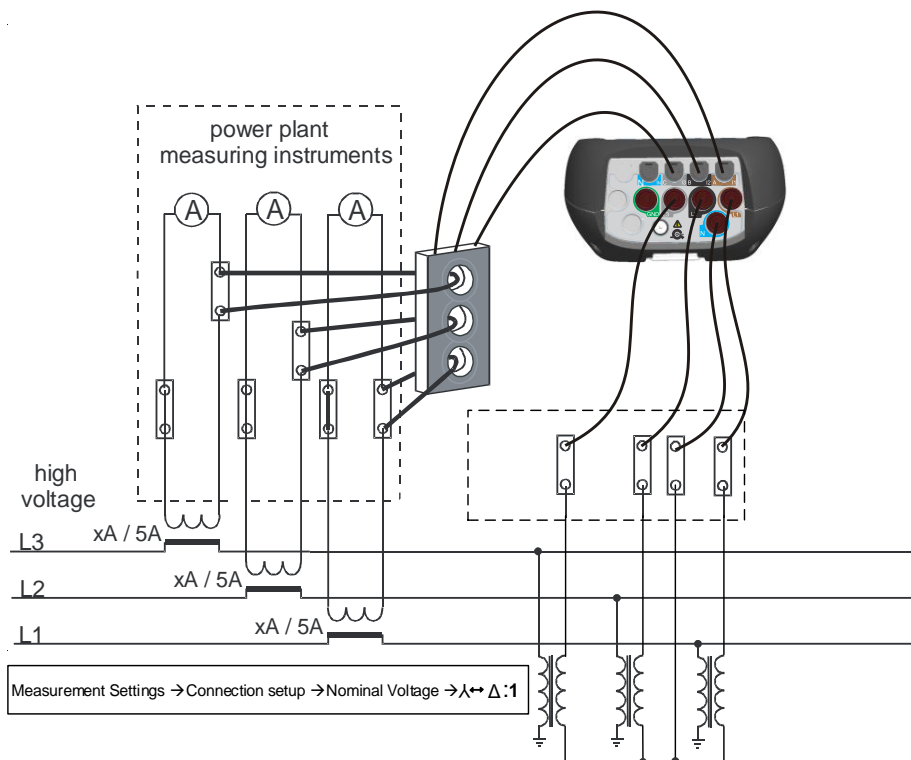
Abbildung 116: Anschließen des Geräts an einen vorhandenen Stromwandler im Mittelspannungssystem (Stern-Stern)
