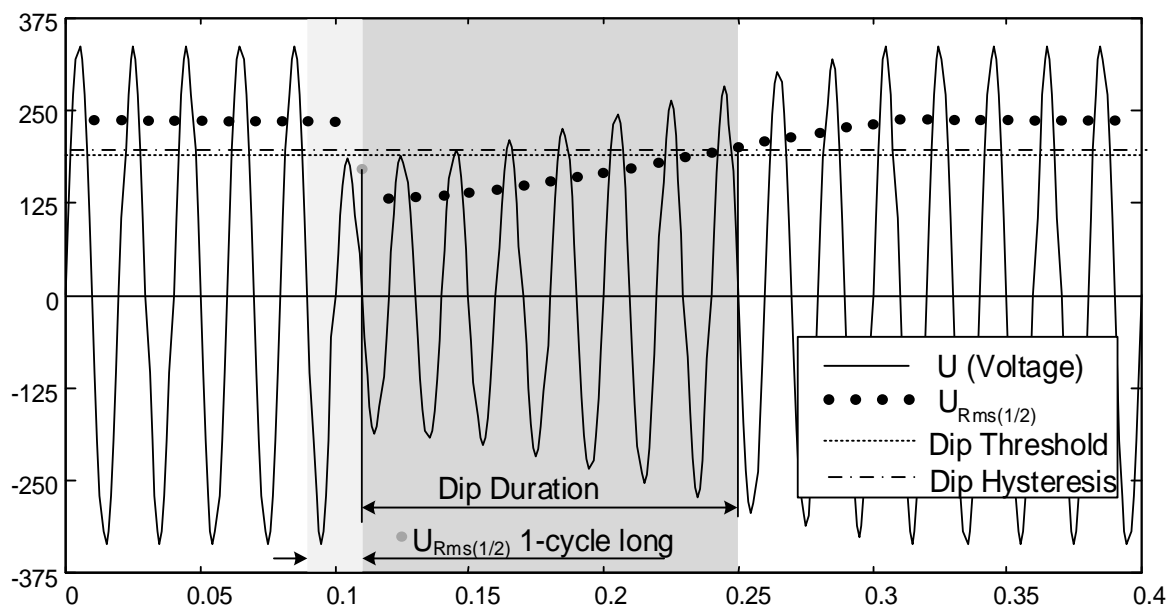
Abbildung 152: U_{Rms(1/2)} 1-Zyklus Messung
