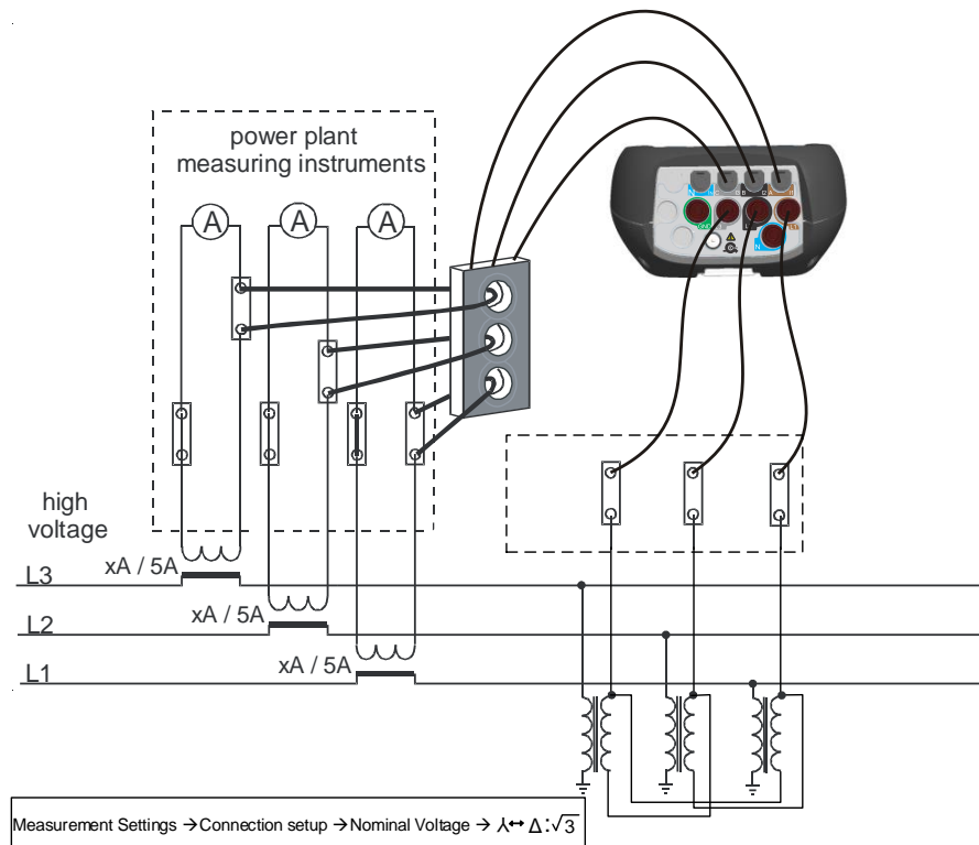
Abbildung 117: Anschließen des Geräts an einen vorhandenen Stromwandler im Mittelspannungssystem (Stern–Dreieck)
