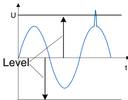
Abbildung 169: Feststellung des Transienten-Auslösers (Niveaualöser)
