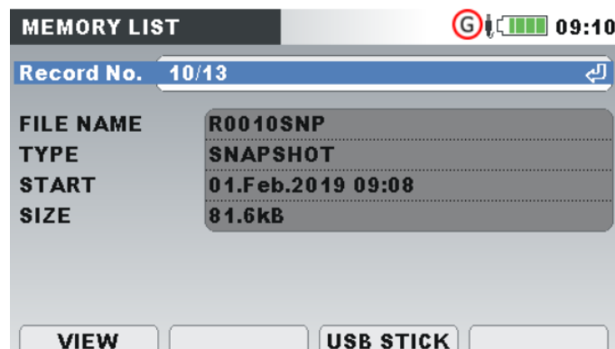
Abbildung 75: Erste Seite der Momentaufnahme im Menü SPEICHERLISTE
