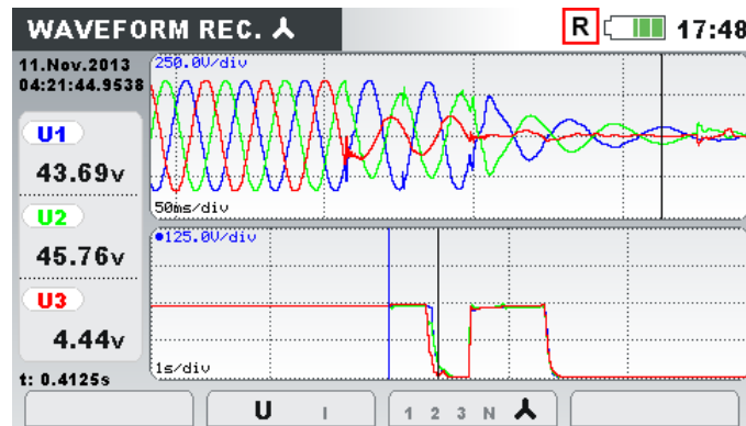
Abbildung 60: Rekorder Bildschirm mit erfasster Wellenform
