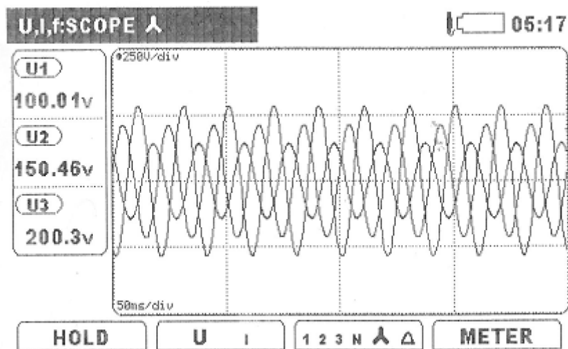
Abbildung 126: BEREICH des Bildschirmausdrucks
