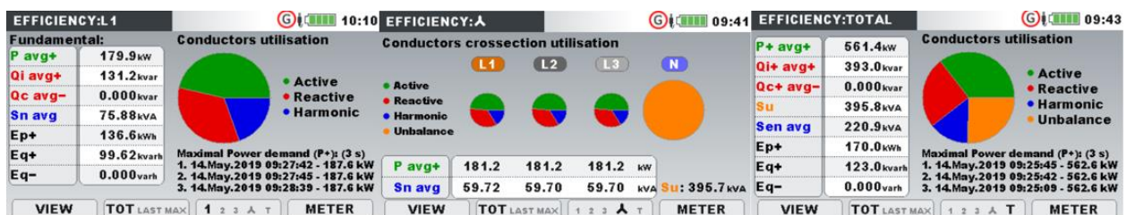
Abbildung 36: Bildschirm Energieeffizienz
