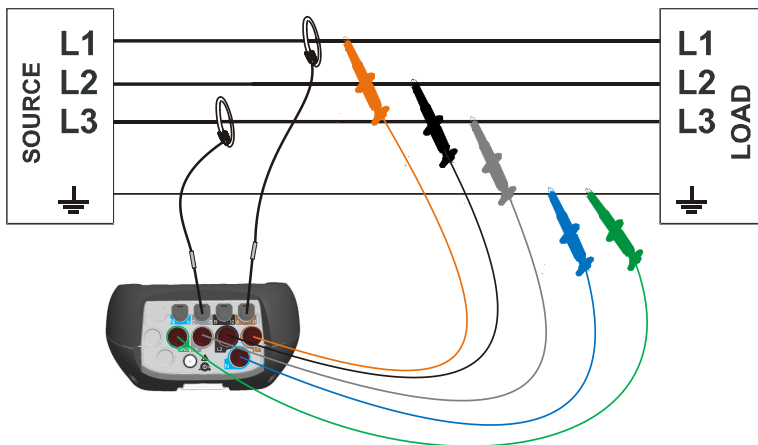
Abbildung 103: Offenes Dreieck-3-Leitersystem (Aronschtaltung)
