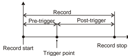
Abbildung 55: Auslösung der Wellenformaufzeichnung
