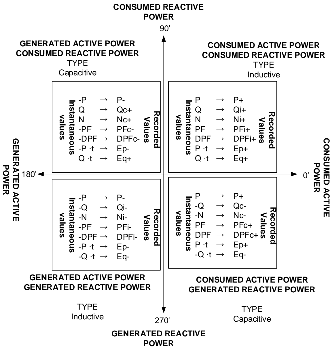
Abbildung 159: Phasen-/Polaritätsdiagramm zu Verbraucht/Erzeugt und Induktiv/Kapazitiv
