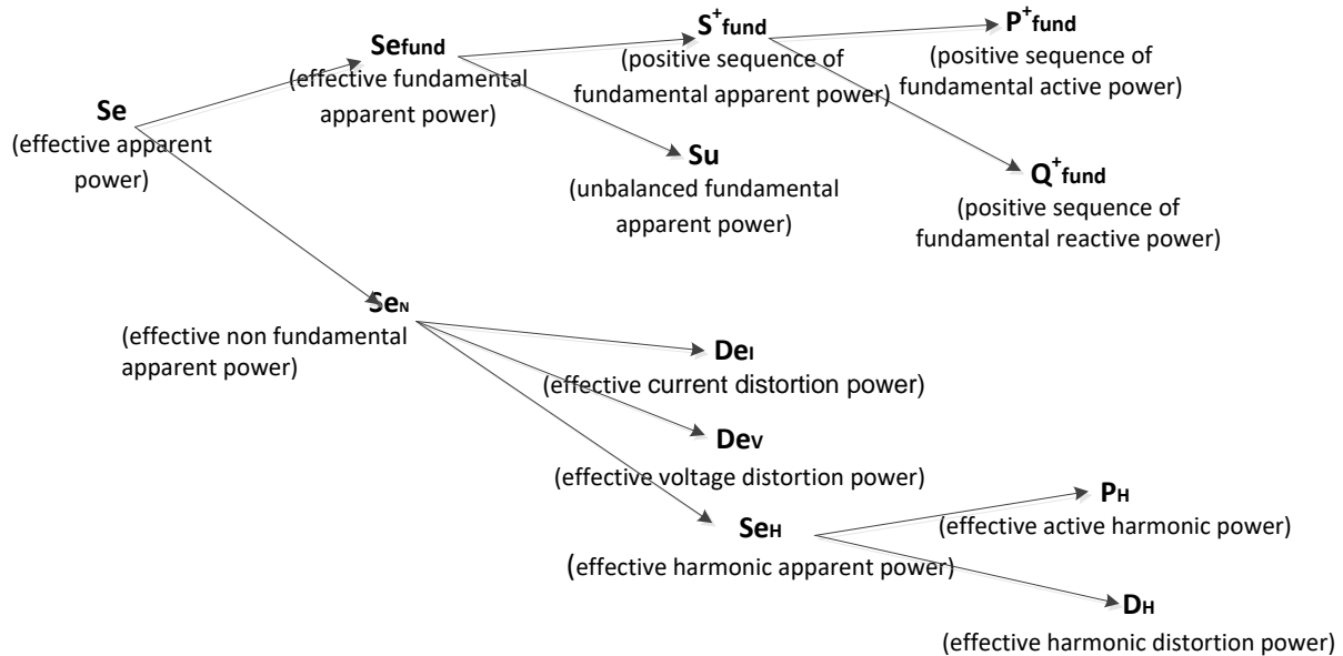
Abbildung 144: IEEE 1459 Organisation der Phasenleistungsmessung (Gesamt)
