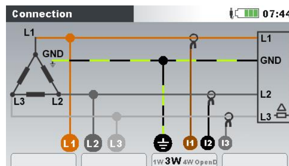
Abbildung 100: Auswählen des 3-Phasen 3-Leitersystems auf dem Gerät
