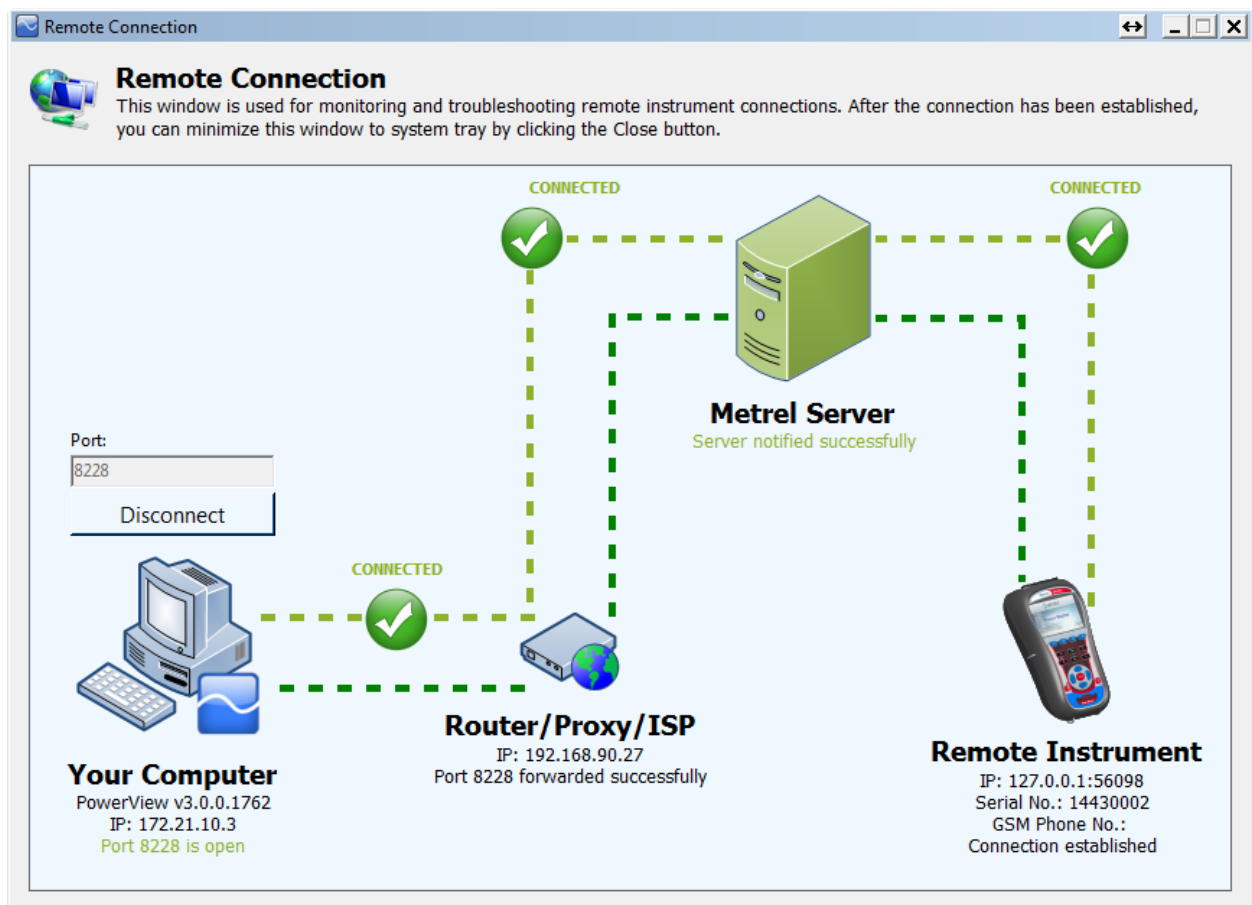
Abbildung 133: Verbindung des Remote-Geräts mit PowerView v.3.0 hergestellt (Schritt 4)
