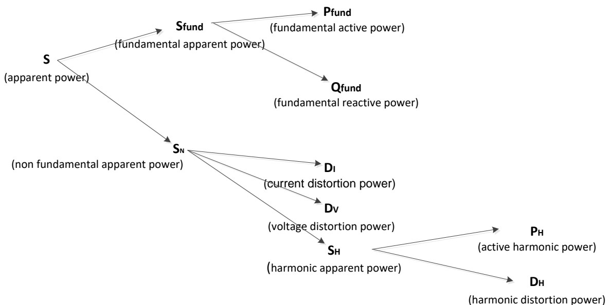
Abbildung 143: IEEE 1459 Organisation der Phasenleistungsmessung (Phase)
