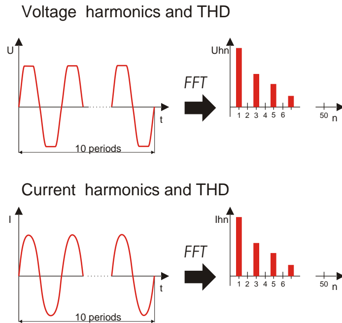
Abbildung 149: Strom- und Spannungsharmonische
