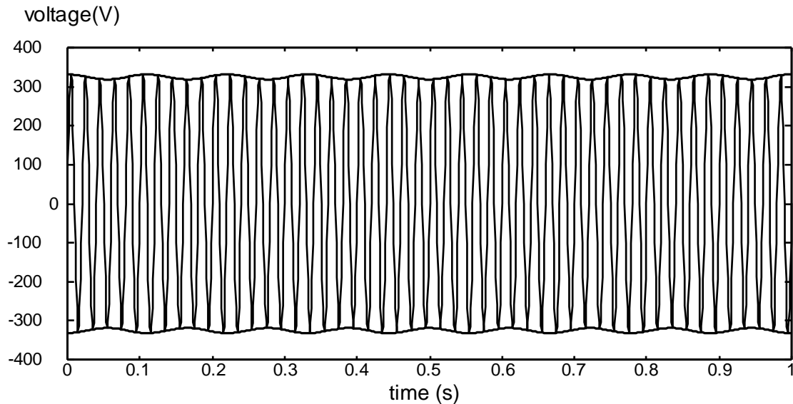
Abbildung 151: Spannungsschwankung
