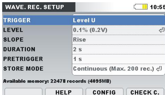
Abbildung 56: Bildschirm mit den Einstellungen des Wellenform-Rekorders
