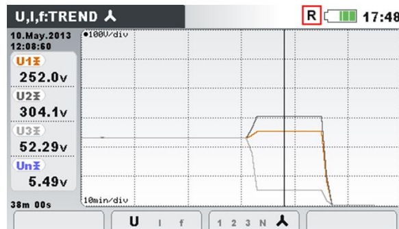
Abbildung 74: Ansicht der Rekorder Daten für den U,I,f-TREND
