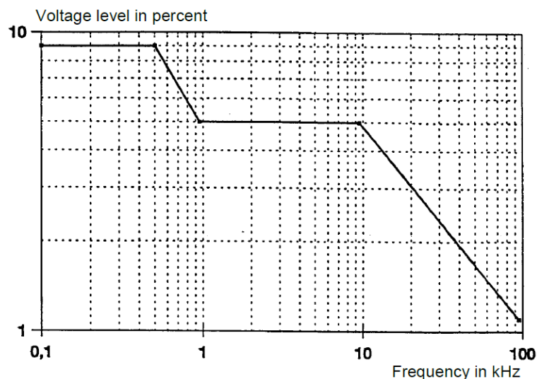
Abbildung 170: Spannungsgrenzwerte bei der Signalübertragung im Versorgungsnetz gemäß EN50160
