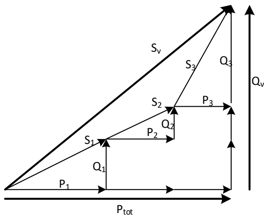
Abbildung 145: Vektorielle Darstellung der Gesamtleistungsrechnung
