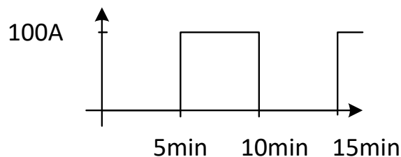
Abbildung 158: Avg Im Vergleich zu Avgon, Schaltlaststrom
