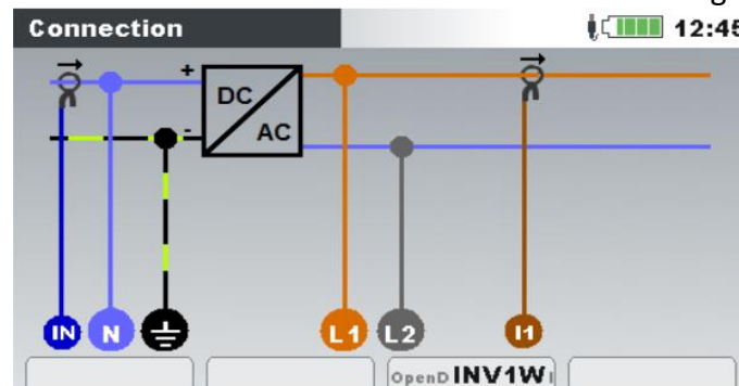
Abbildung 108: Auswählen des einphasigen Wechselrichtersystems auf dem Gerät
