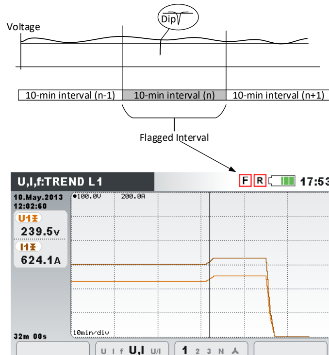
Abbildung 160: Markierte Daten zeigen, dass der aggregierte Wert unzuverlässig sein könnte
