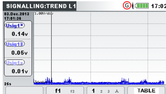
Abbildung 52: Bildschirm mit dem Trend der Netzsignale
