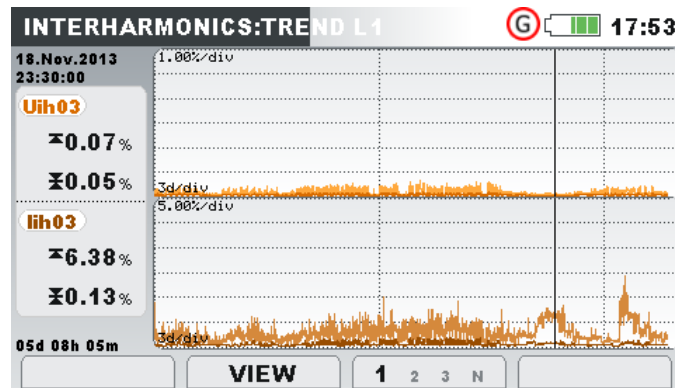
Abbildung 41: Bildschirm mit dem Trend der Harmonischen und Zwischenharmonischen
