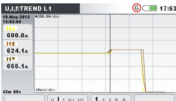
Abbildung 26: Trends aller Ströme
