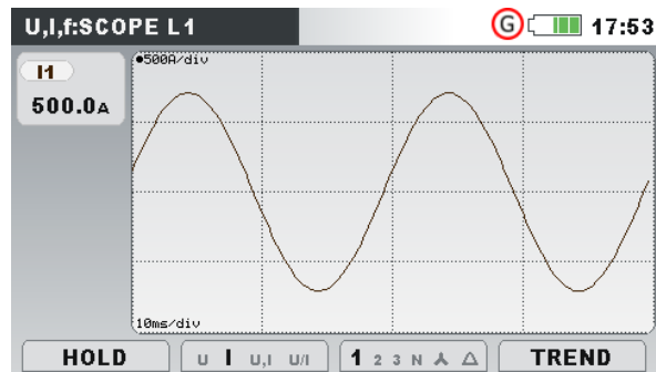
Abbildung 19: Nur Wellenform des Stroms
