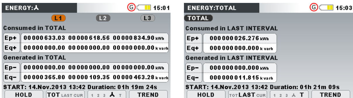
Abbildung 34: Bildschirm mit den Energiezählern
