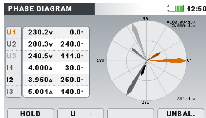
Abbildung 44: Bildschirm des Phasendiagramms
