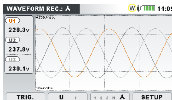
Abbildung 59: Oszilloskop-Bildschirm des Wellenform-Rekorders
