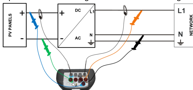
Abbildung 109: Einphasiges Wechselrichtersystem
