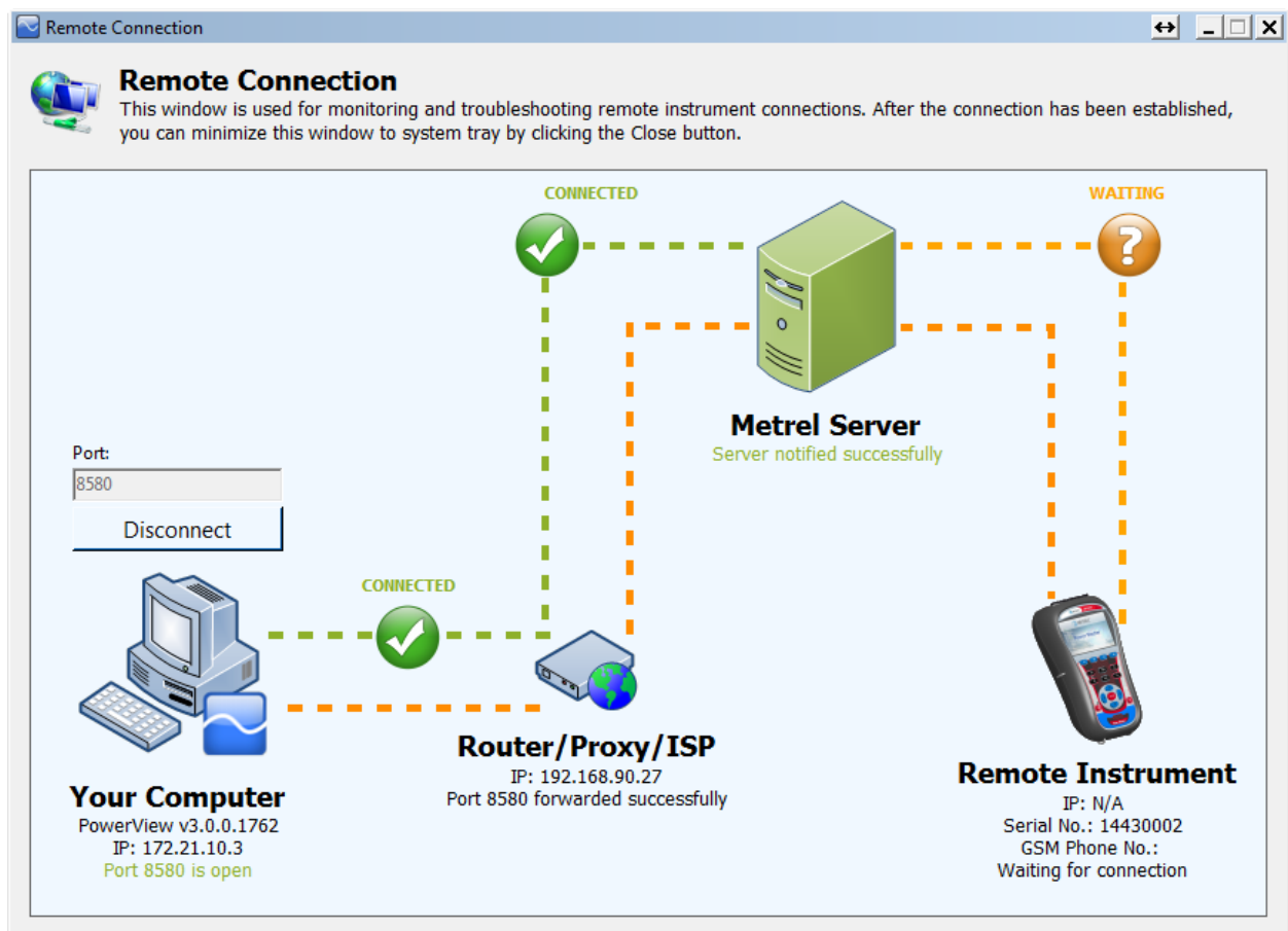
Abbildung 131: PowerView-Verbindung zum LAN- und Metrel-Server hergestellt (Schritte 1 und 2)
