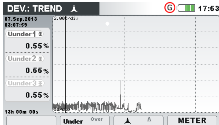
Abbildung 50: Unterabweichung und Überabweichung auf dem (TREND)-Bildschirm
