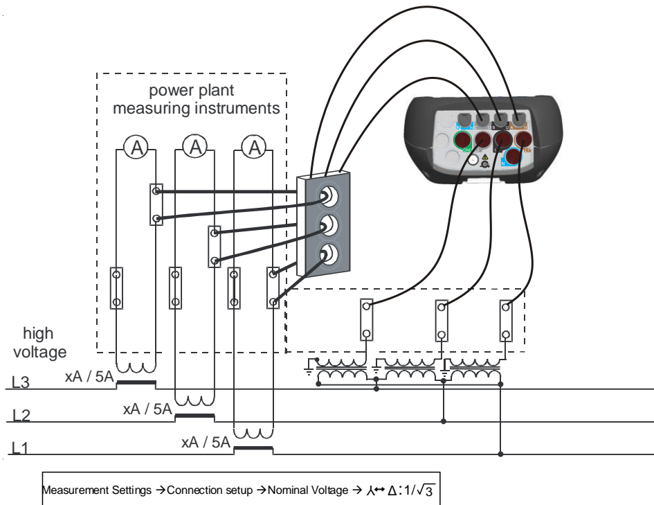
Abbildung 115: Anschließen des Geräts an einen vorhandenen Stromwandler im Mittelspannungssystem (Dreieck-Stern)
