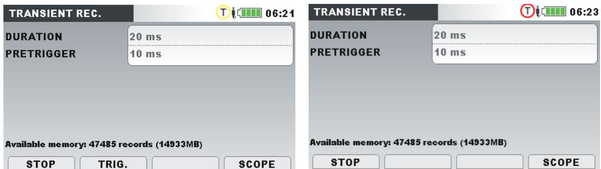
Abbildung 64: Transientenrekorder-Erfassungsbildschirm (Wartephase/Aufzeichnung) – MI 2892/MI 2885
