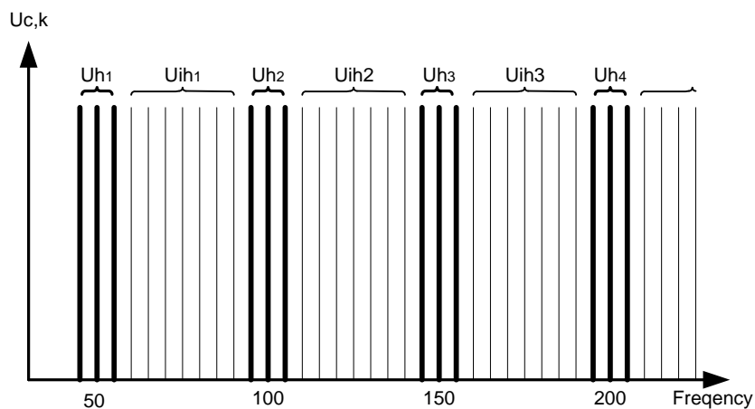
Abbildung 150: Darstellung der Untergruppe von Harmonischen / Zwischenharmonischen für eine 50-Hz-Versorgung
