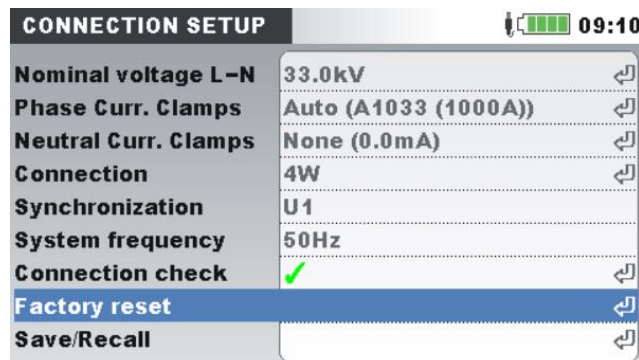
Abbildung 97: Menü Anschlusseinstellung
