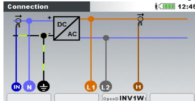
Abbildung 110: Auswählen des dreiphasigen Wechselrichtersystems auf dem Gerät
