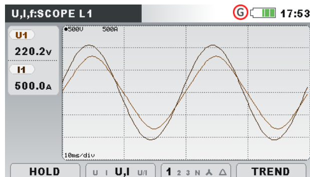
Abbildung 20: Spannungs- und Stromwellenform (Einzel-Modus)
