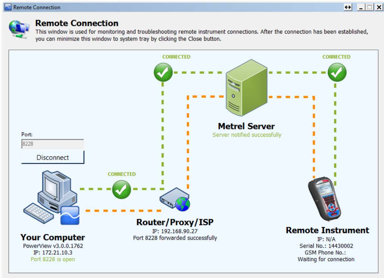
Abbildung 132: Remote-Verbindung des Geräts zum Metrel-Server hergestellt (Schritt 3)
