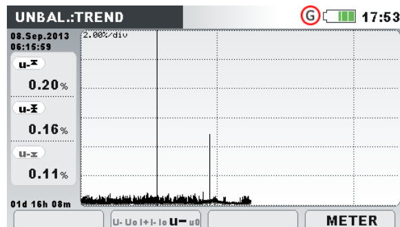
Abbildung 46: Bildschirm mit dem Symmetrietrend
