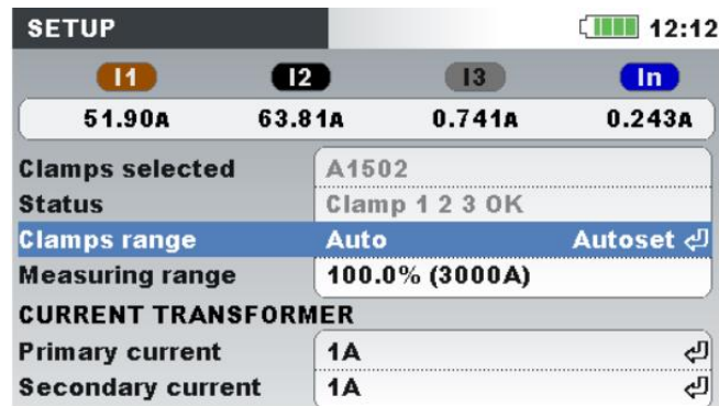
Abbildung 118: Automatische Bereichswahl Smart- Stromzangen
