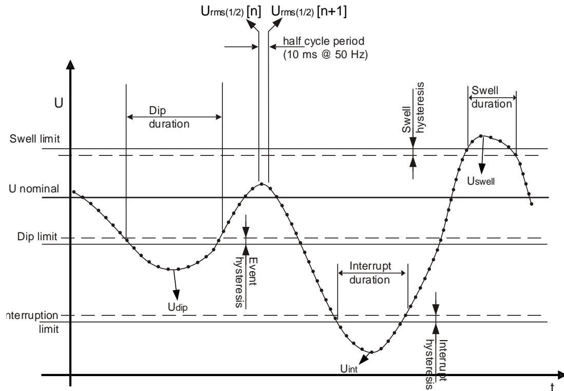
Abbildung 153: Definition der Spannungsereignisse
