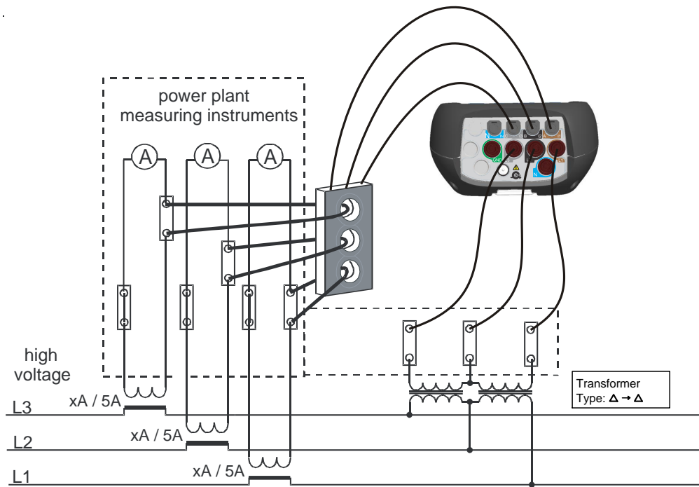
Abbildung 113: Anschließen des Geräts an einen vorhandenen Stromwandler im Mittelspannungssystem (Aron / offenes Dreieck)
