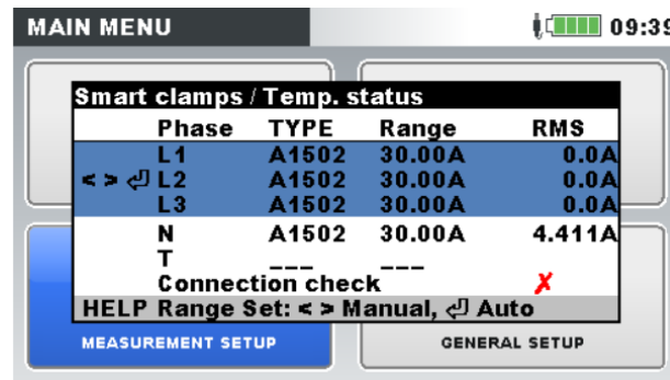
Abbildung 123: Automatisch erkannter Stromzangenstatus
