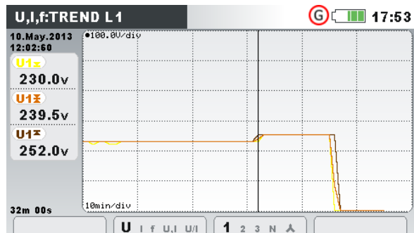
Abbildung 23: Spannungstrend (einzelne Spannung)
