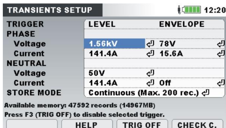
Abbildung 61: Bildschirm mit den Einstellungen des Wellenform-Rekorders – MI2893
