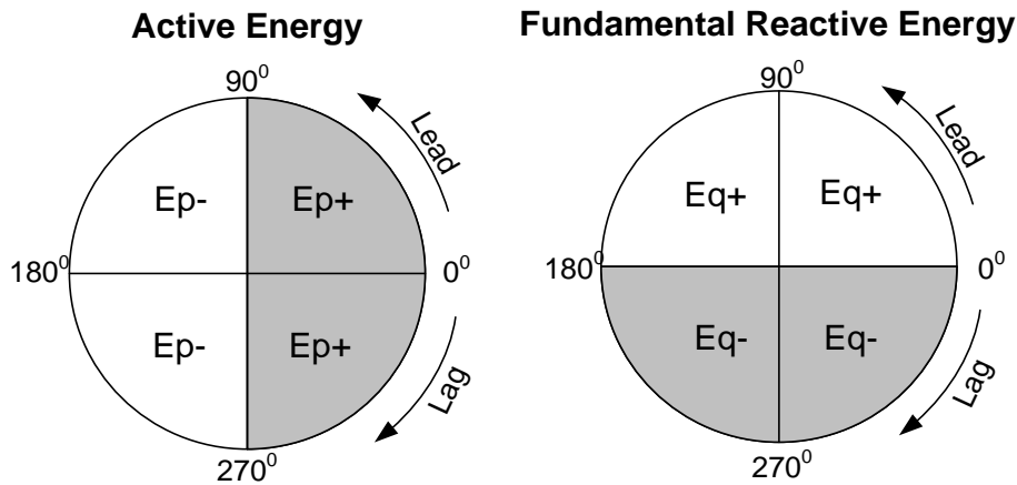
Abbildung 147: Energiezähler und Quadrantenverhältnis
