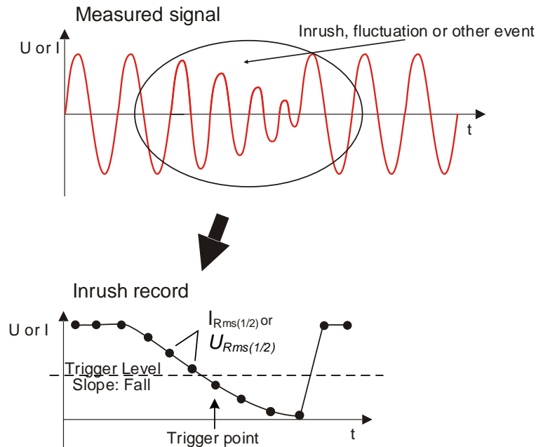
Abbildung 166: Niveaualösung
