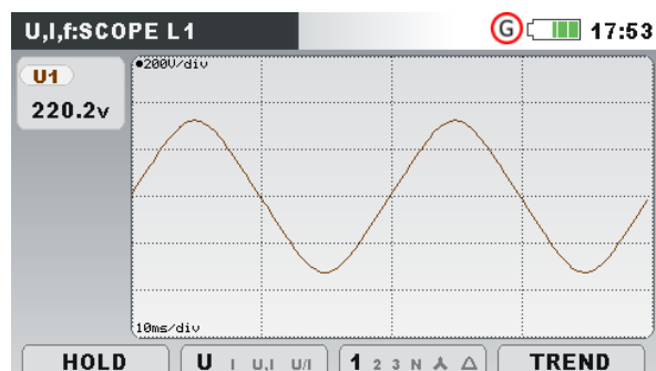
Abbildung 18: Nur Wellenform der Spannung
