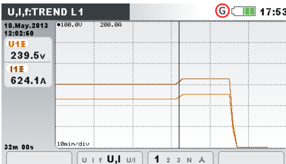
Abbildung 24: Spannungs- und Stromtrend (Einfach-Modus)
