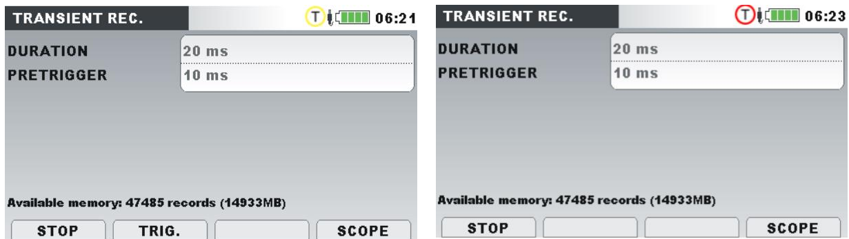
Abbildung 63: Erfassungsbildschirm des Transienten-Rekorders (Wartephase/Aufnahme) – MI 2893
