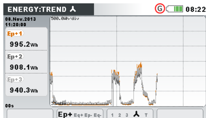
Abbildung 35: Bildschirm Energietrend
