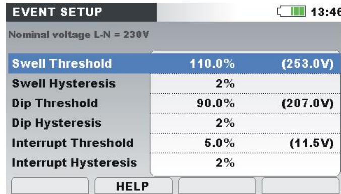
Abbildung 79: Bildschirm für die Ereigniseinrichtung
