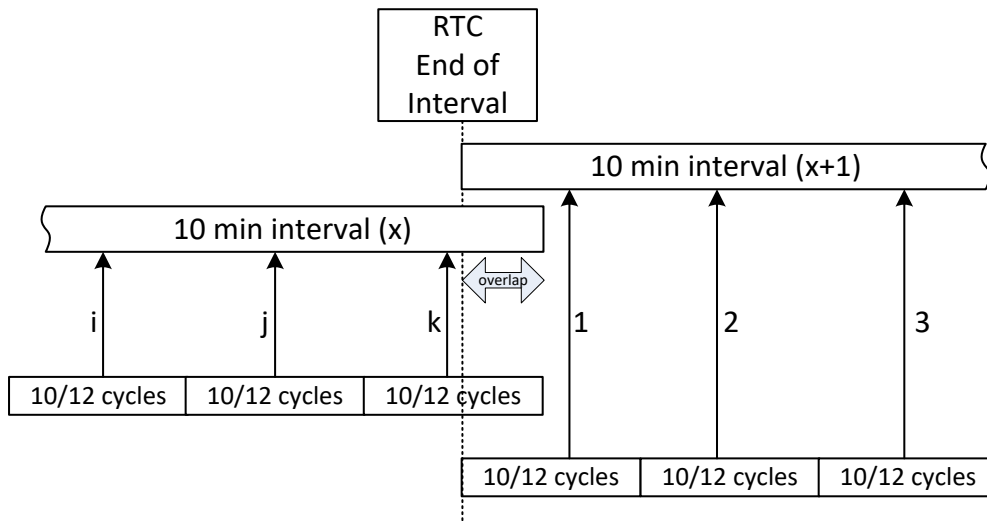
Abbildung 157: Synchronisierung und Aggregation von 10/12-Zyklusintervallen
