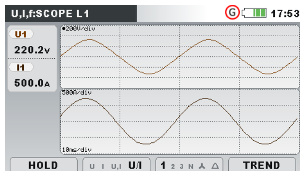
Abbildung 21: Spannungs- und Stromwellenform (Dual-Modus)
