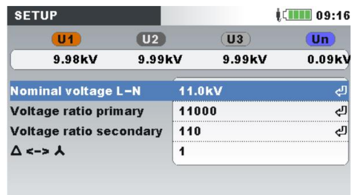
Abbildung 112: Beispiel für das Spannungsverhältnis eines 11-kV- / 110-kV-Wandlers
