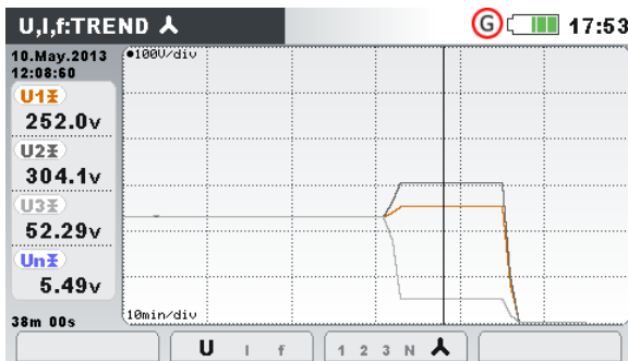
Abbildung 22: Spannungstrend (alle Spannungen)
