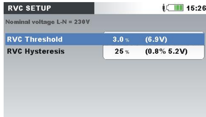
Abbildung 82: RVC-Einstellungsbildschirm
