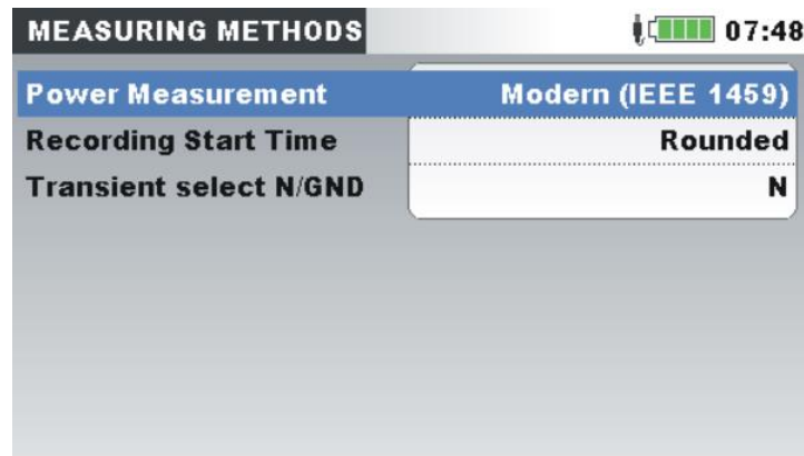
Abbildung 83: Bildschirm Einstellung der Messmethoden – MI 2893
