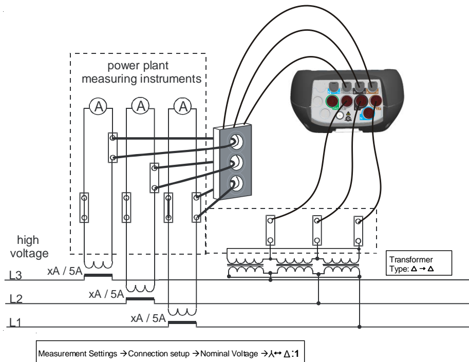
Abbildung 114: Anschließen des Geräts an einen vorhandenen Stromwandler im Mittelspannungssystem (Dreieck–Dreieck)
