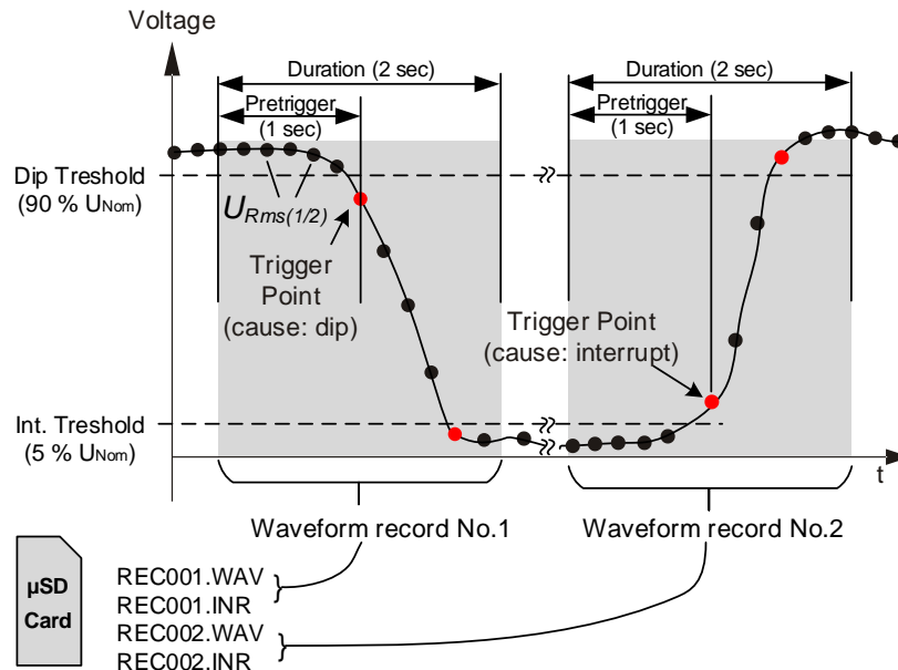
Abbildung 162: Spannungs-Ereignis-Auslösung
