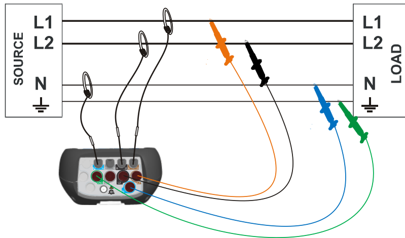
Abbildung 107: 2-Phasen 4-Leitersystem
