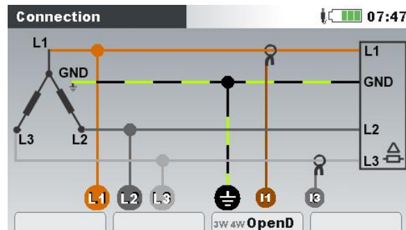
Abbildung 102: Auswählen des offenen Dreieck-3-Leitersystems auf dem Gerät
