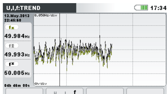
Abbildung 27: Frequenztrend
