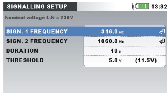
Abbildung 81: Bildschirm zur Netzsignaleinrichtung
