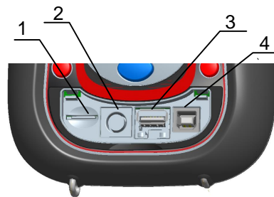
Abbildung 5: Seitliches Anschlussfeld
