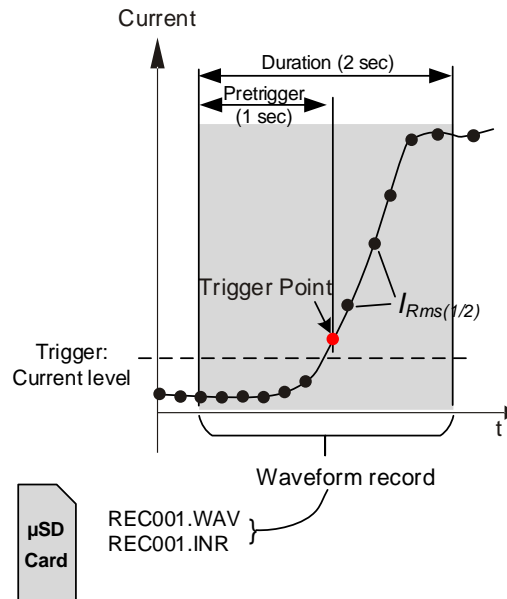
Abbildung 164: Strom-Niveau-Auslösung (Einschaltspitzen)
