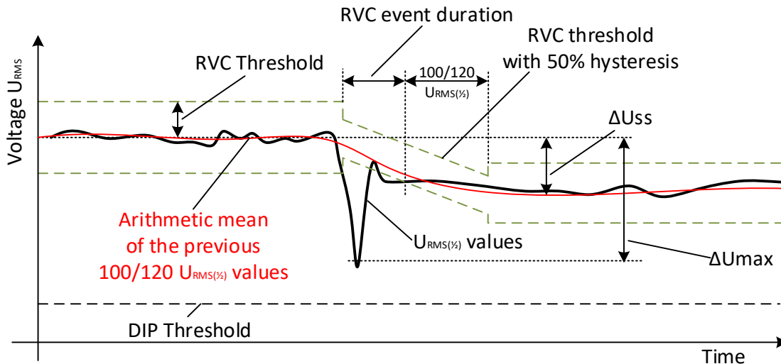
Abbildung 156: RVC-Ereignisbeschreibung
