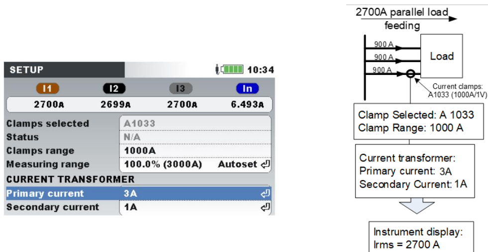
Abbildung 119: Parallele Einspeisung bei großen Lasten
