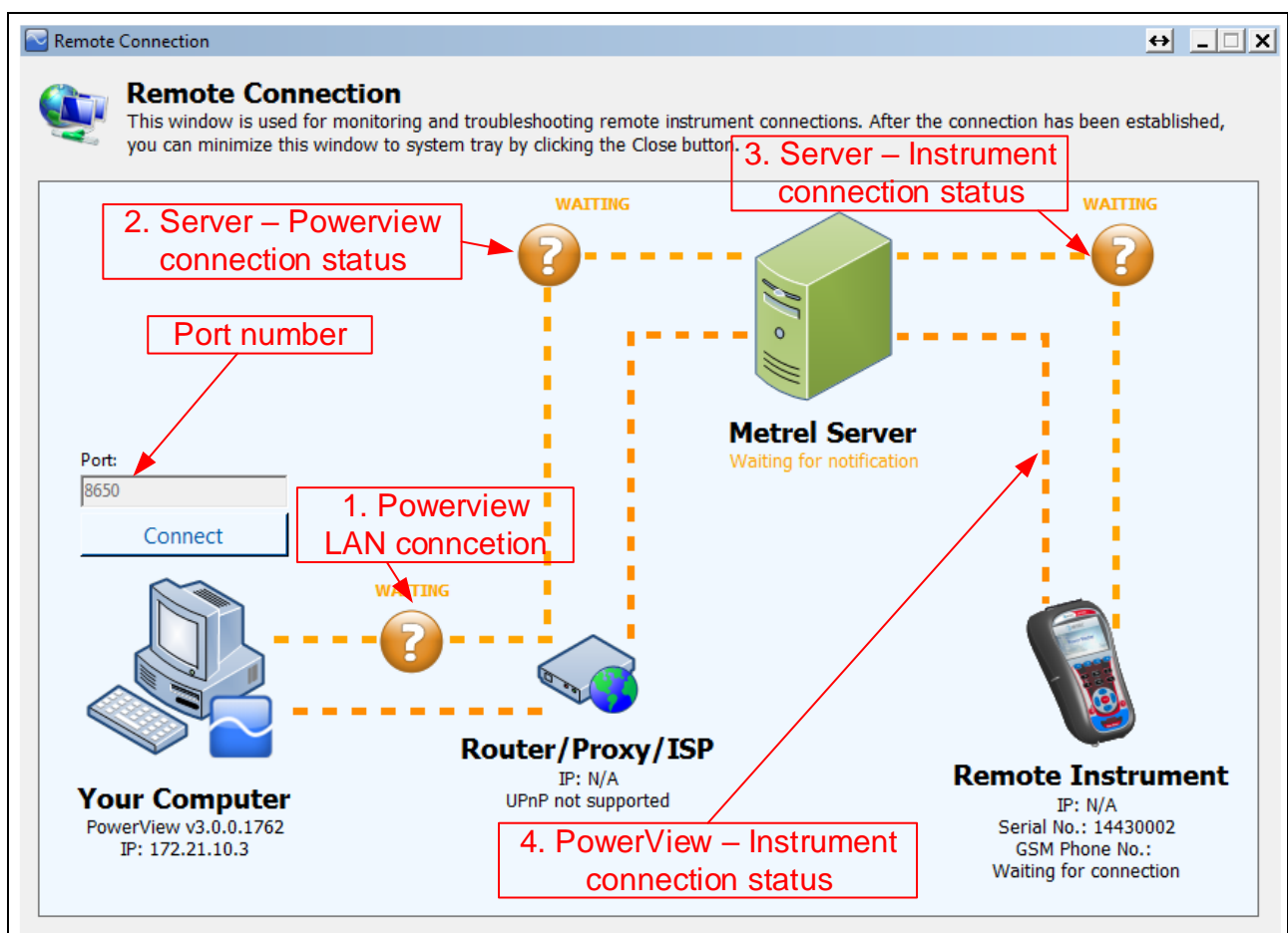
Abbildung 130: Remote-Verbindungsmonitor von PowerView v3.0
