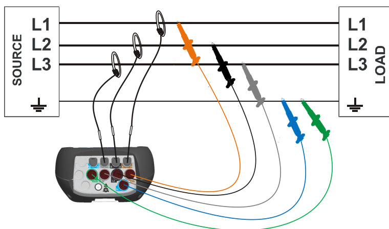
Abbildung 101: 3-Phasen 3-Leitersystem
