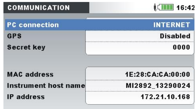
Abbildung 128: Bildschirm zur Einrichtung der Internetverbindung
