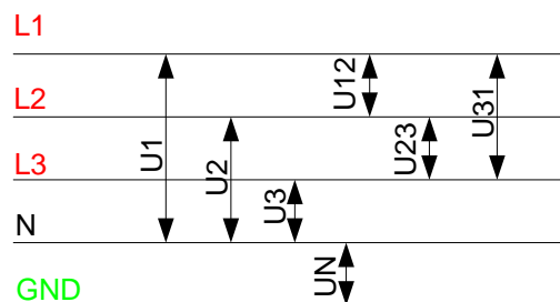
Abbildung 142: Phasen- und Phase-Phase-(Leiter)-Spannung
