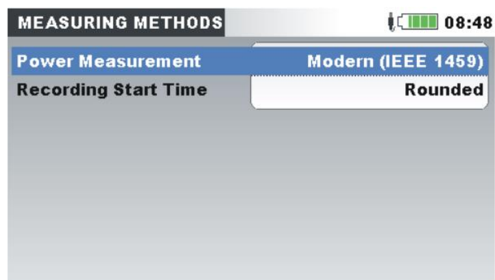
Abbildung 84: Bildschirm Einstellung der Messmethoden – MI 2892/MI 2885
