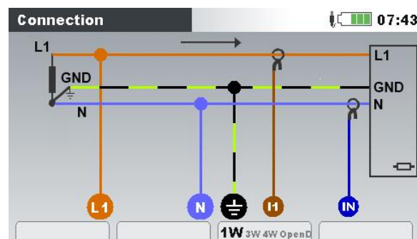
Abbildung 104: Auswählen des 1-Phasen 3-Leitersystems auf dem Gerät
