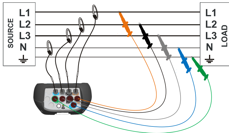
Abbildung 99: 3-Phasen 4-Leitersystem
