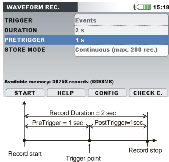
Abbildung 161: Darstellung der Auslösung und Vorauslösung
