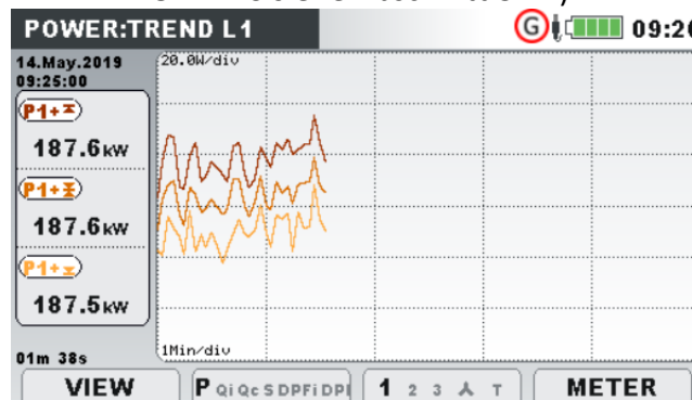
Abbildung 33: Bildschirm Leistungstrend
