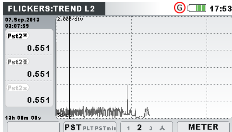
Abbildung 43: Bildschirm mit dem Flickertrend
