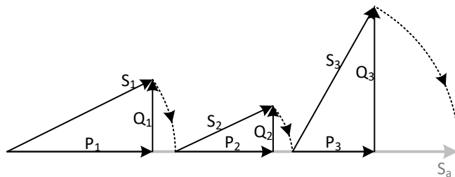
Abbildung 146: Arithmetische Darstellung der Gesamtleistungsrechnung
